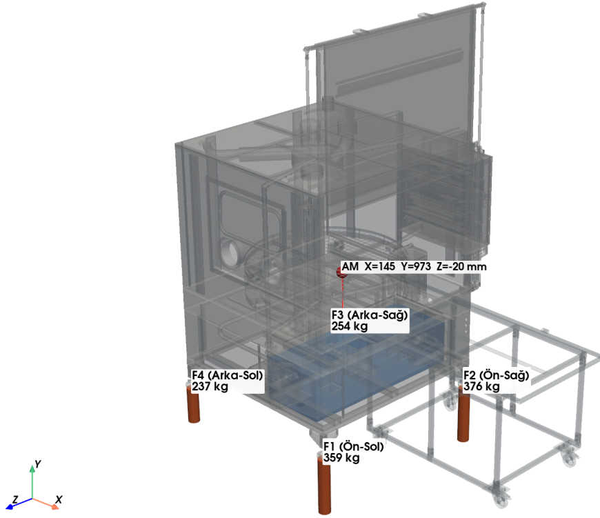
Şekil 7. Senaryo C (su + 300 kg sepet yükü, 1.226 kg).
